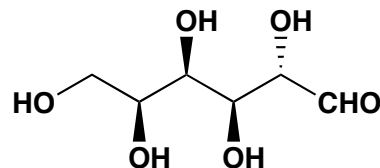
L-Gulose
