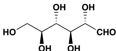
L-Allose
