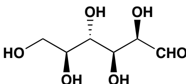
L-Altrose
