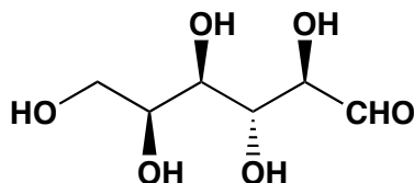
L-Talose
