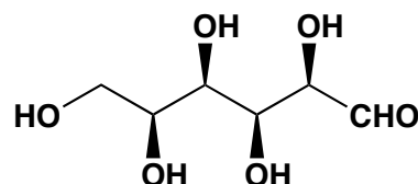
L-Idose
