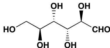
L-Mannose
