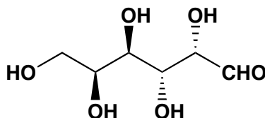
L-Galactose
