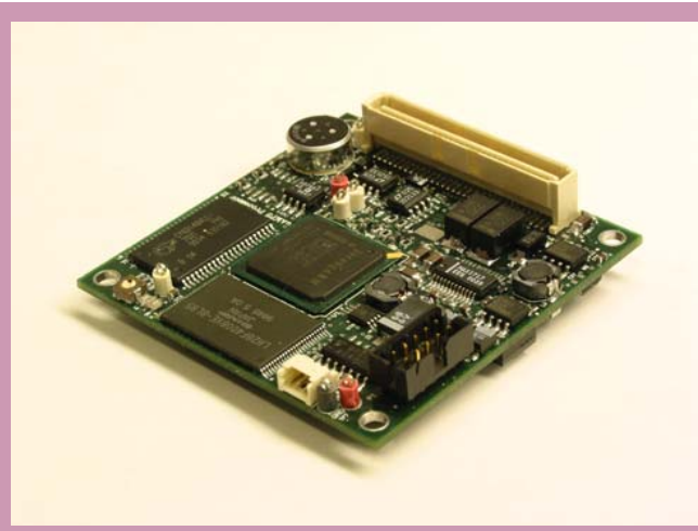
206MHz StrongARM
