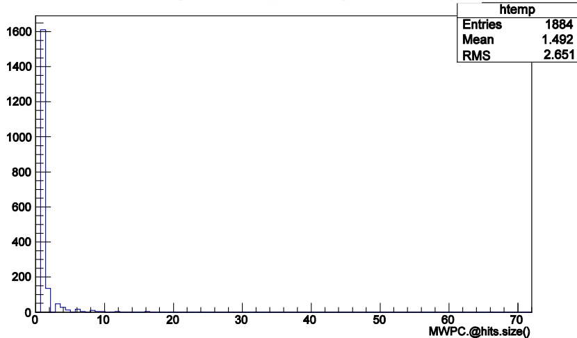
MWPC.@hits.size() {MWPC.@hits.size() != 0}
