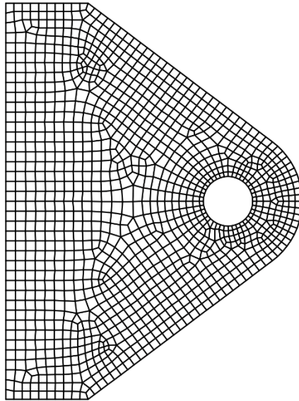
(d) The mesh of 4-node elements with incompatible modes
