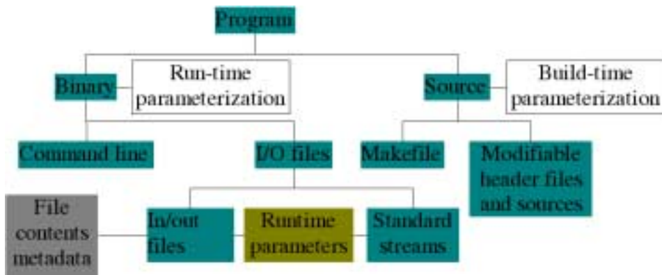
Fig. 12. Hierarchy of schemata
