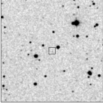
POSS-II R
