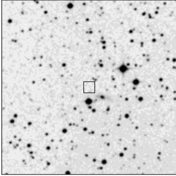
AAO R
